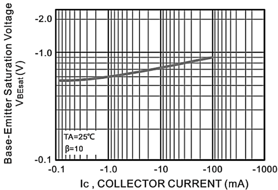
Fig.5 V_{BEsat} \text{--} I_c
