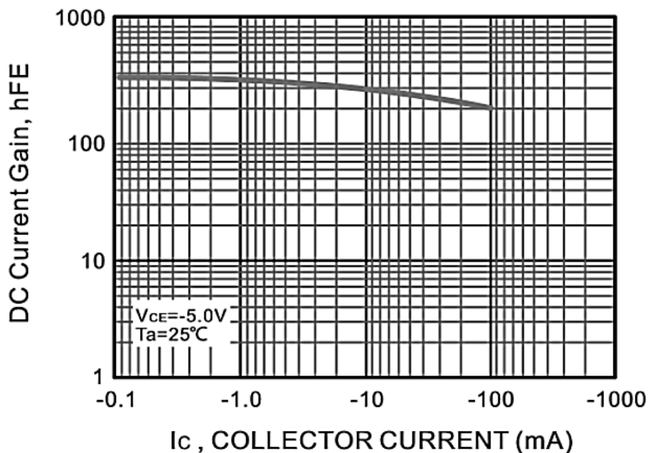
Fig.3 h_{FE} -- I_c
