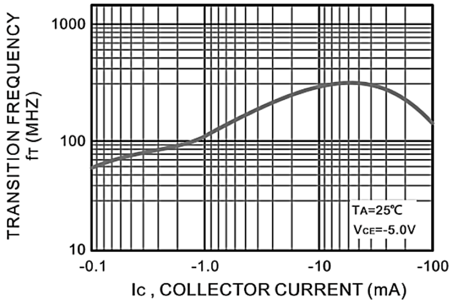
Fig.7 f_t -- I_c
