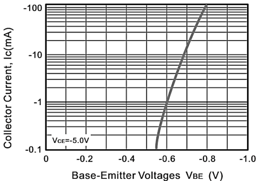
Fig.4 I_c -- V_{BE}
